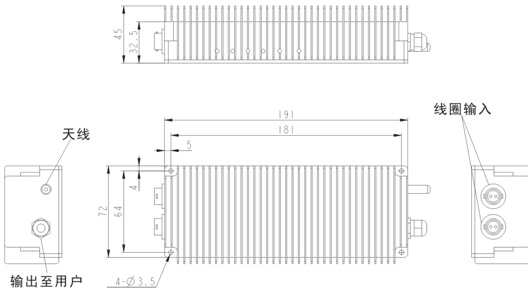
图 4.接收控制器尺寸及接口说明
