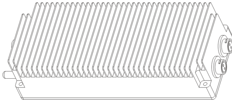
图 5.接收控制器外形尺寸
